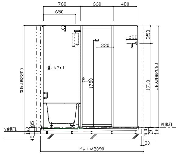
[C] 展開図
