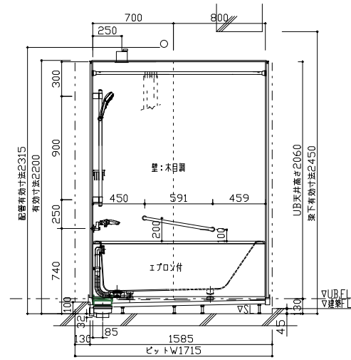
[B] 展開図
