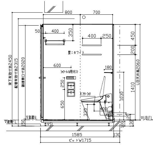
[D] 展開図
