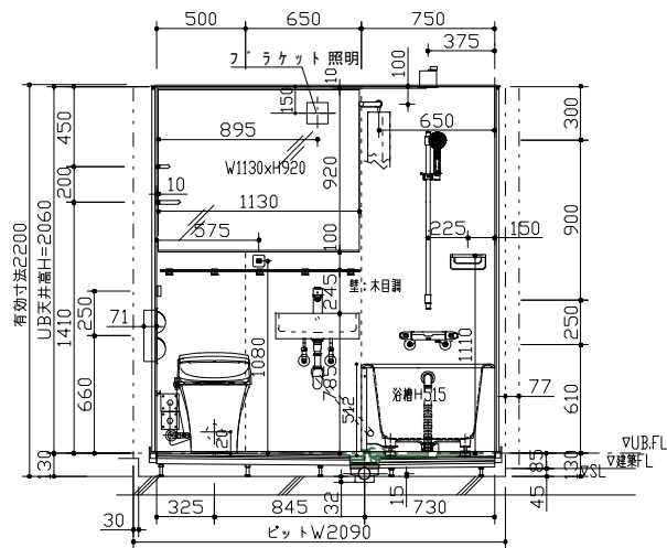
[A] 展開図
