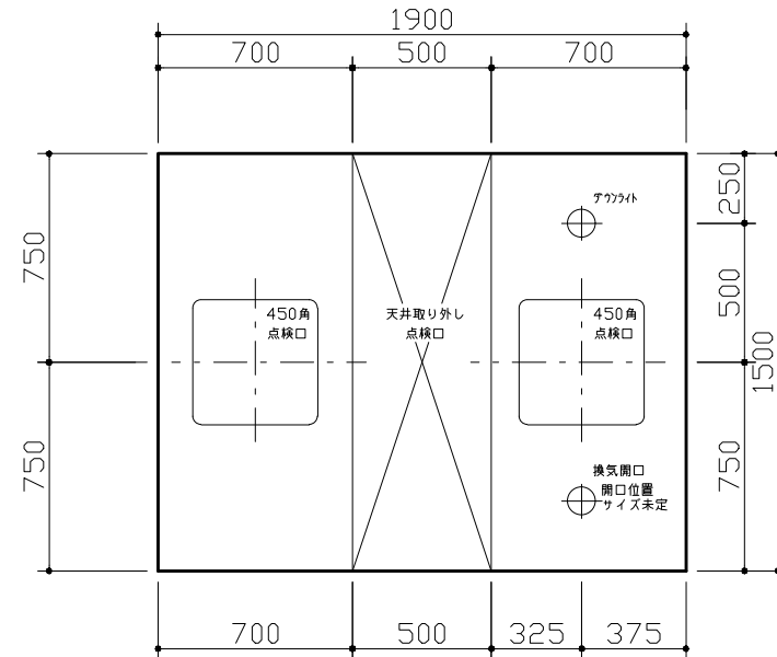
[天井伏図]
