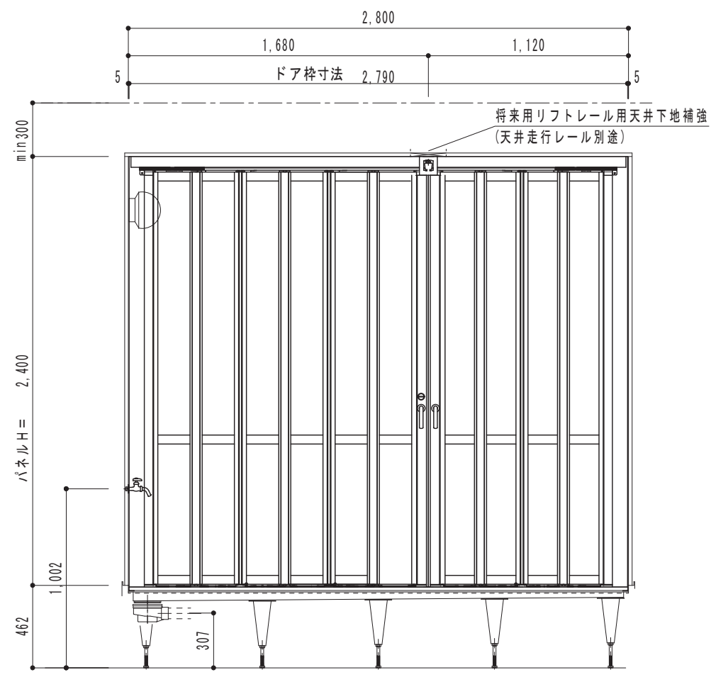
【C展開図】
