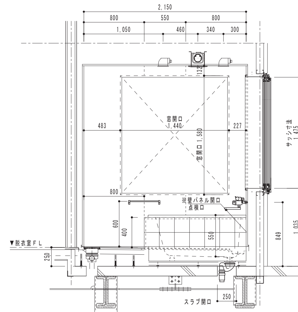
【D展開図】
