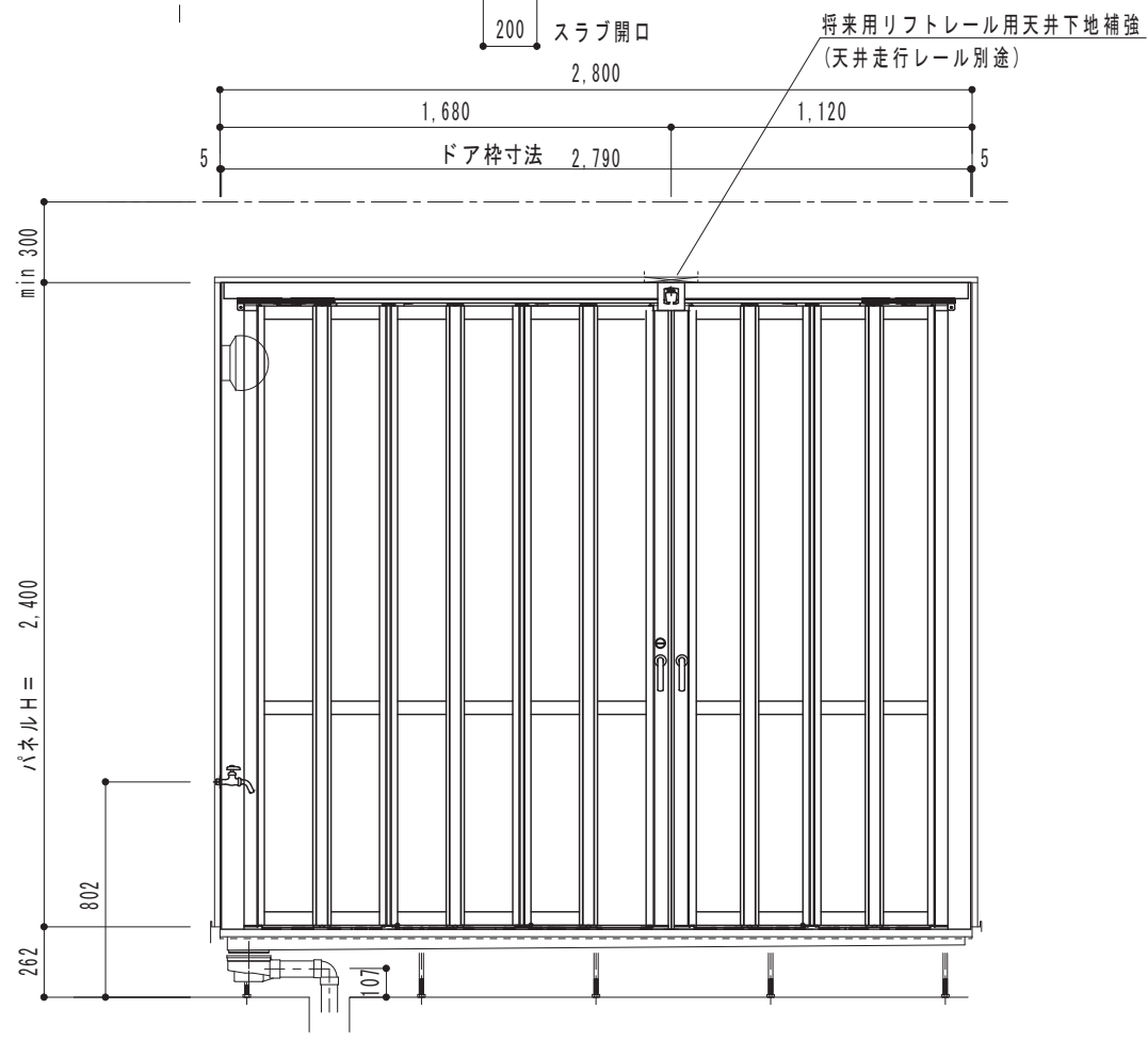
【C展開図】
