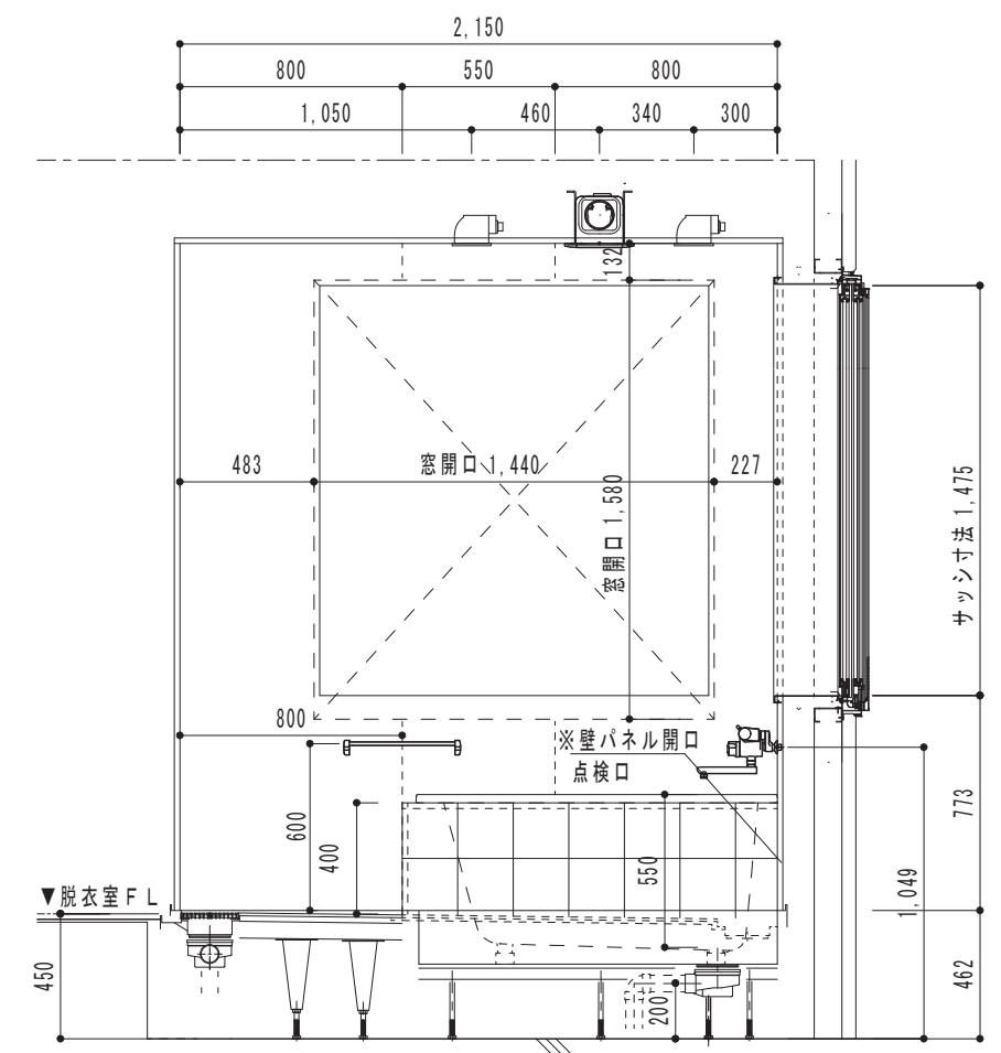
【D展開図】
