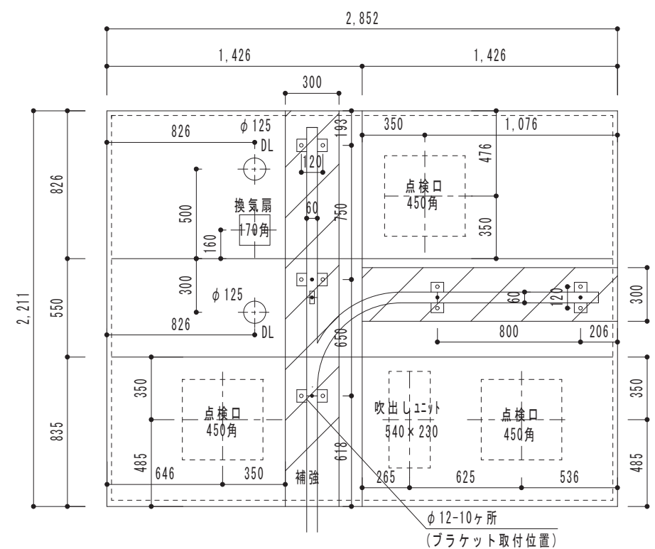
【 天井伏せ図 1/30 】
