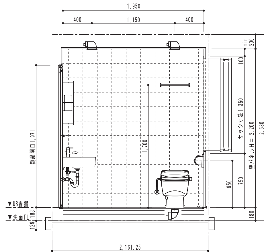
[D展開図]
