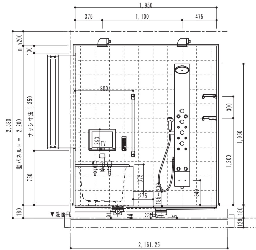
[B展開図]
