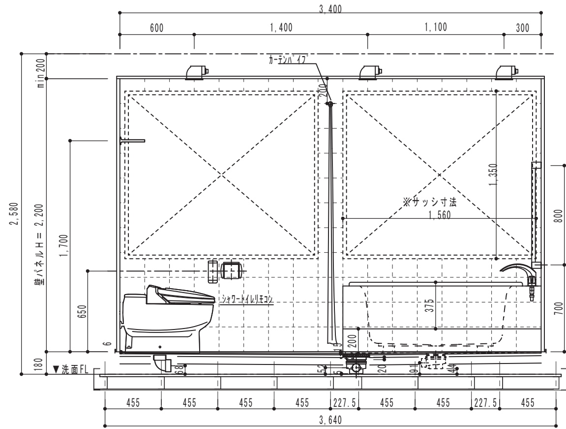
[A展開図]
