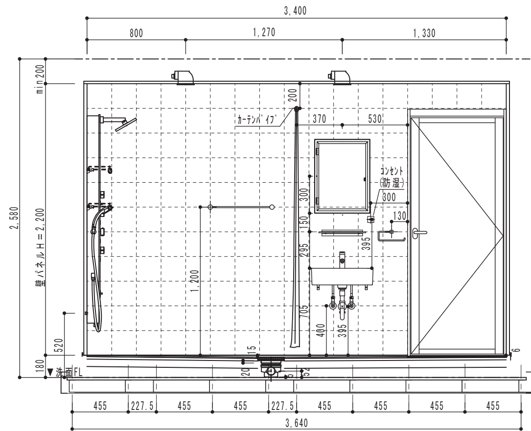
[C展開図]
