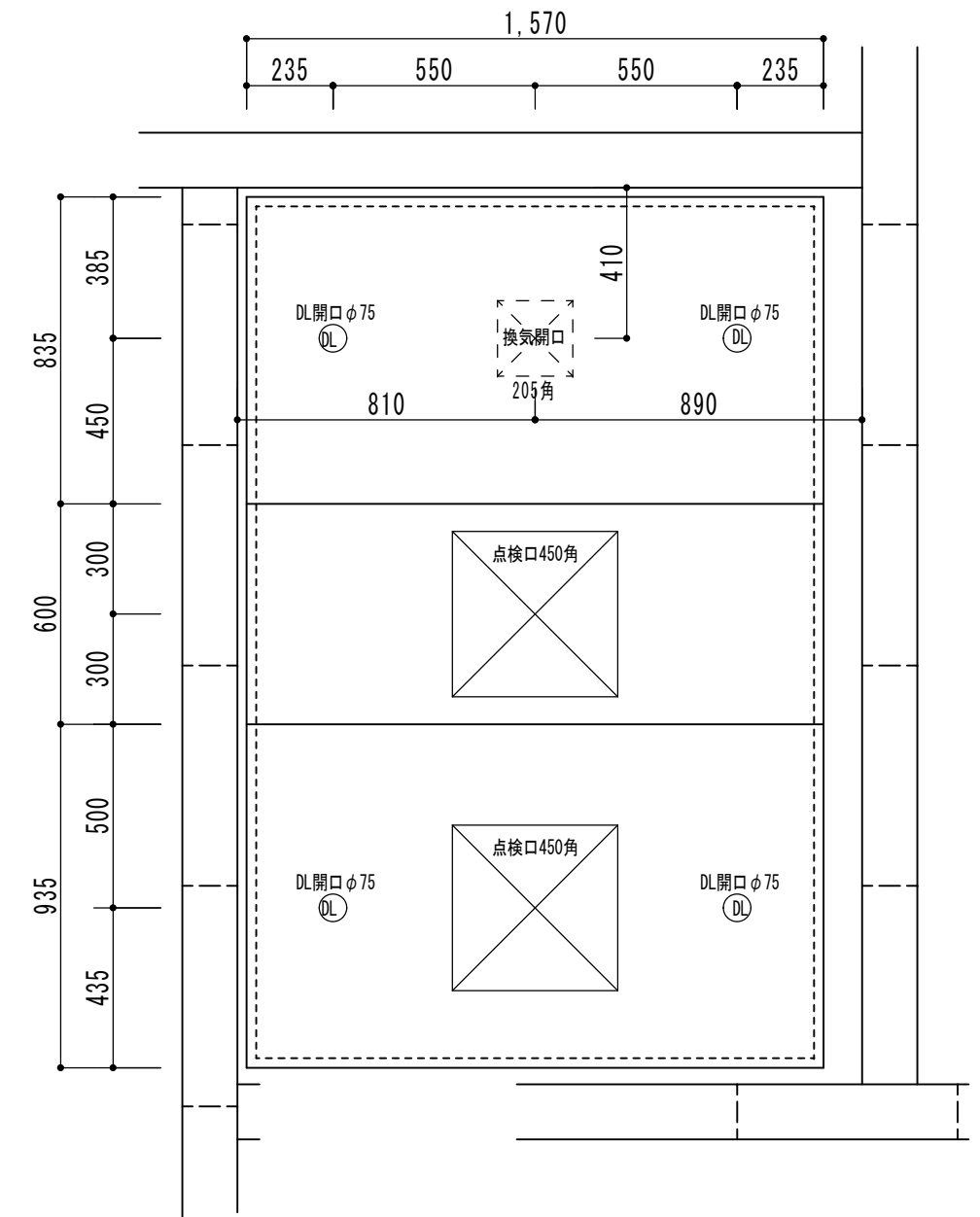
【天井伏図】
