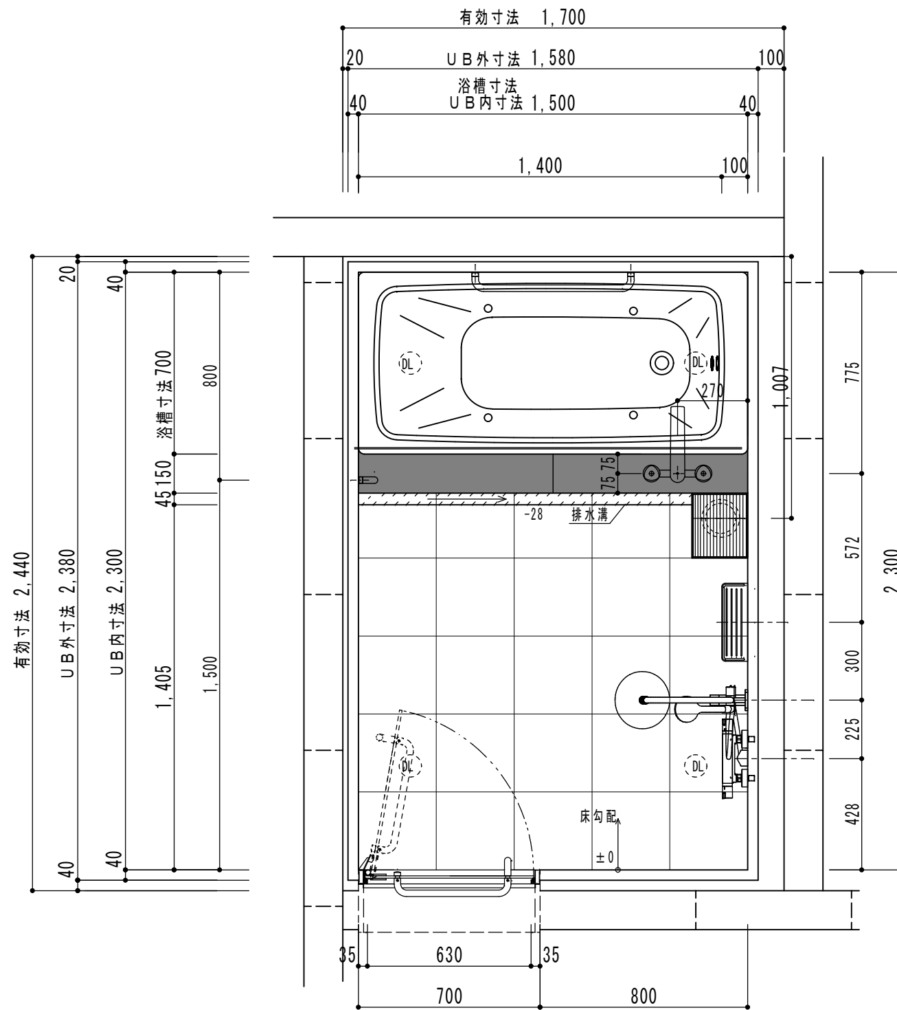
【平面図】
